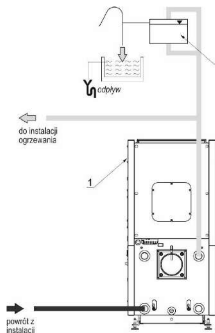
Rysunek 5. Przykładowy schemat zabezpieczeń kotła BIO SLIM: 1-kocioł; 2-otwarte naczynie wzbiorcze.
