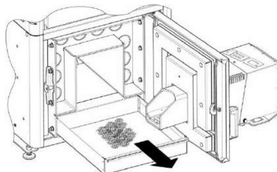
KROK 6. Usunąć nagromadzony popiół i pył
