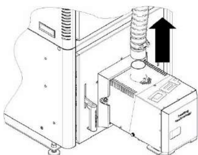
KROK 1. Zdemontować elastyczną rurę zsyłu paliwa.
