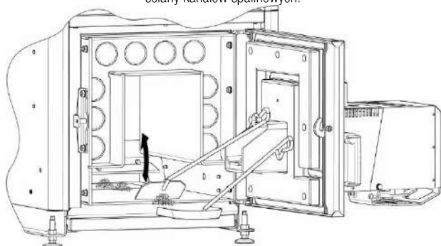
KROK 10. Po wysunięciu szuflady na popiół, odchylić klapę przegrody i wygarnąć nagromadzony popiół.
