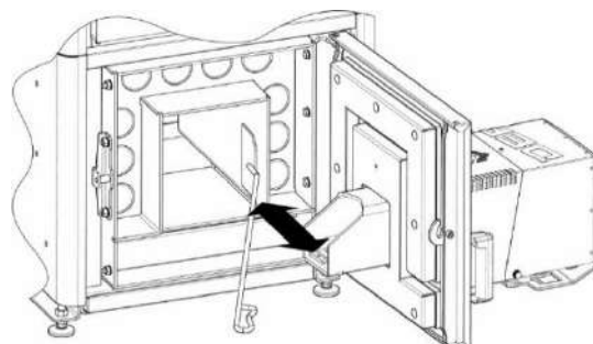
KROK 5. Za pomocą dostarczonych narzędzi oczyścić płomienicę
