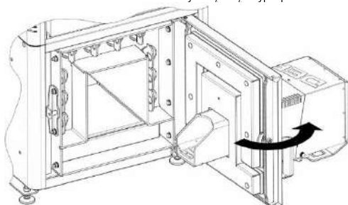
KROK 2. Otworzyć drzwi kotła.
