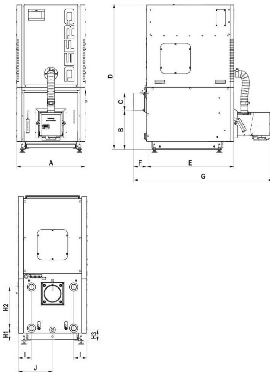
Rysunek 1. Podstawowe wymiary kotła CALORI.
