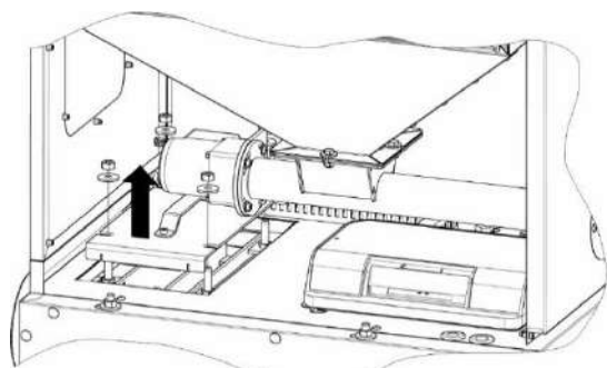
KROK 8. Odkręcić śruby mocujące wyczystkę i zdjąć pokrywę wyczystki.
