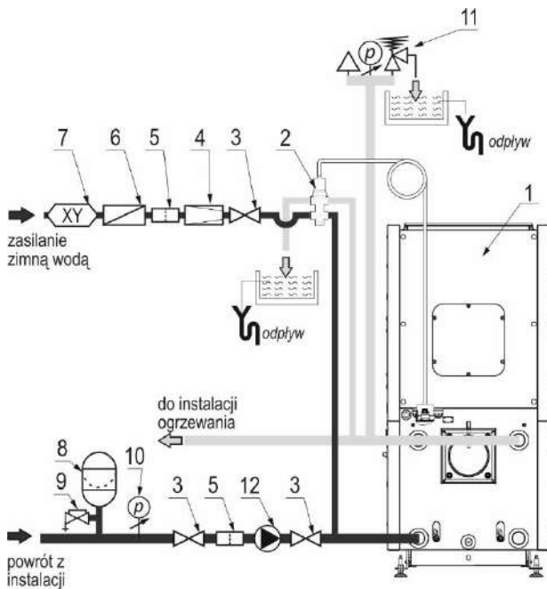
Rysunek 7. Przykładowy schemat zabezpieczeń kotła w układzie zamkniętym: 1-kocioł; 2-zabezpieczenie termiczne przed przegrzaniem /np. zawór 544/; 3-czujnik temperatury z kapilarą; 4-zawór zwrotny; 5-filtr wody użytkowej; 6-armatura bezpieczeństwa; 7-naczynie przeponowe; 8-zawór kołpakowy; 9-manometr.
