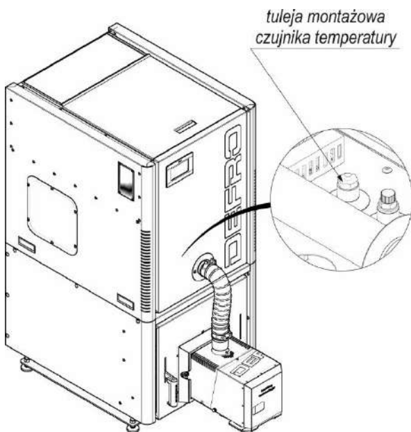
Rysunek 6. Umieszczenie tulei czujnika temperatury.
