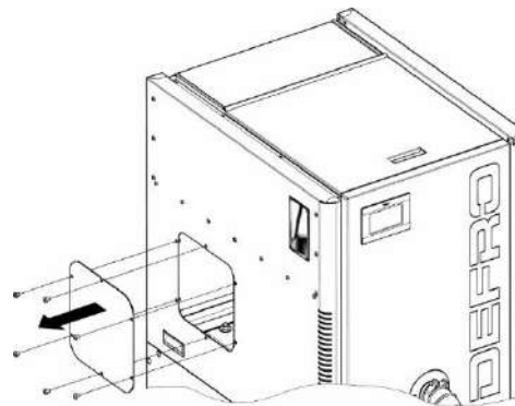
KROK 7. Odkręcić wkręty mocujące pokrywę rewizyjną i zdjąć pokrywę.
