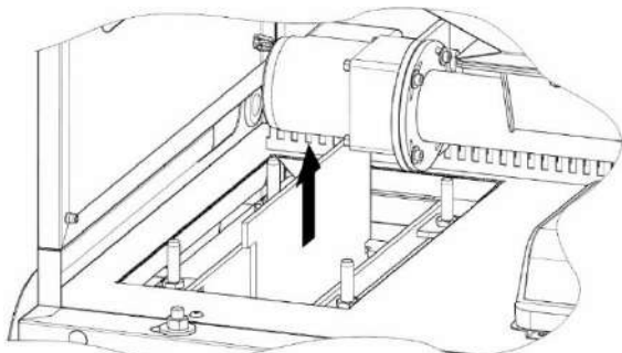
KROK 9. Wysunąć przegrodę kanału spalinowego i oczyścić. Oczyścić także ściany kanałów spalinowych.
