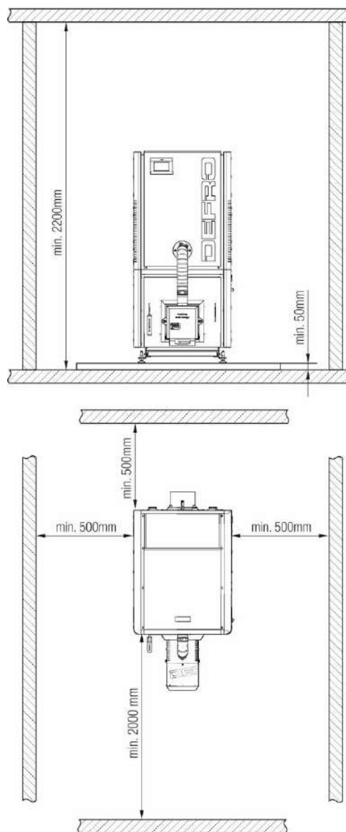
Rysunek 4. Ustawienie kotła w pomieszczeniu kotłowni.
